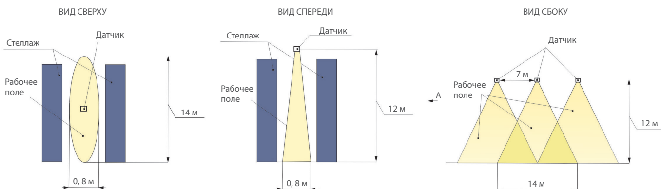
Рабочая зона светильника с датчиком
